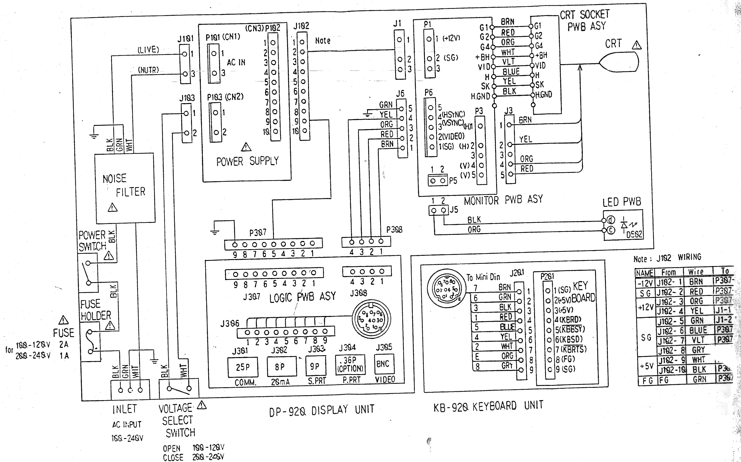
FIG. 10-1 VG-920 WIRING
