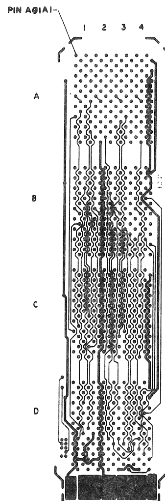
LAYER 1
