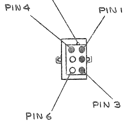
VIEW A-A WIRING SIDE SCALE: NONE
